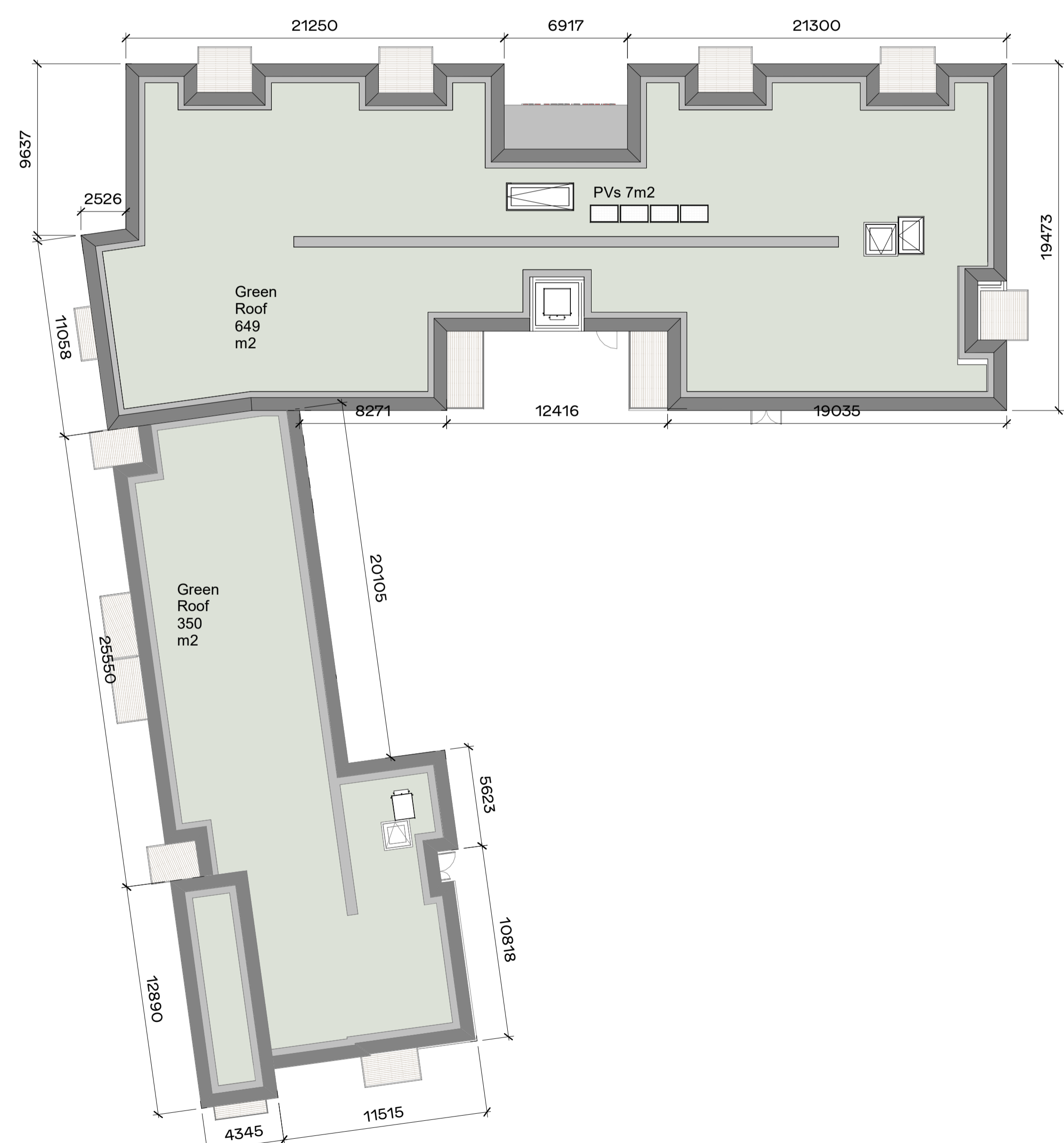
1 1200_BG4_BLOCKPLAN_L04_RF_FFL 1 : 200
